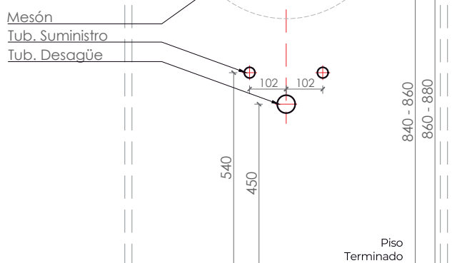
INSTALACIÓN FRONTAL ESC. 1:10
